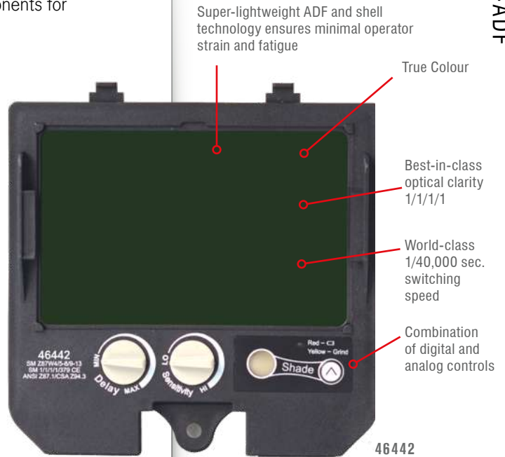
455 Digital/Analog ADF
